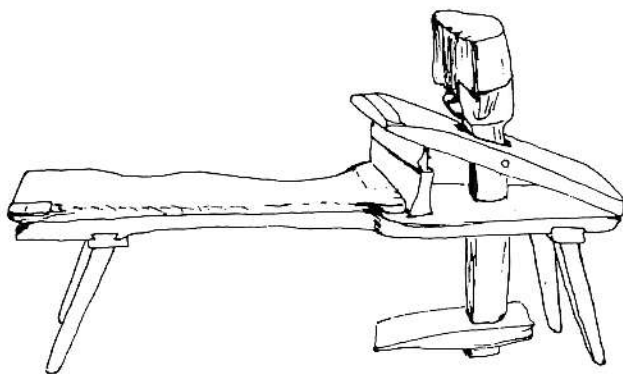
Tunnbindarens skärbänk. Teckning av Åsa Ljungström. Efter Hantverk i Sverige (1989).
